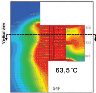
Рис. 7. Пример тепловых полей вокруг наружных блоков при CFD-моделировании. Вид сверху. Для наружных блоков этого производителя допустимая температура составляет 50 °C
