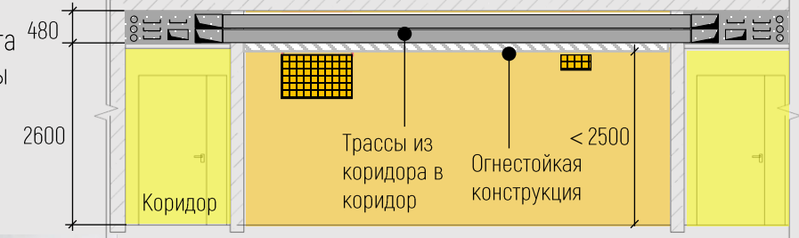
Разрез. Стало
