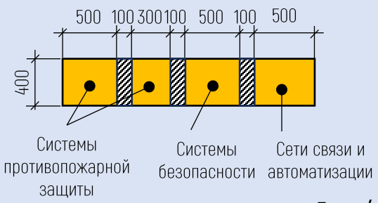
Шахты для одного коридора жилого этажа
