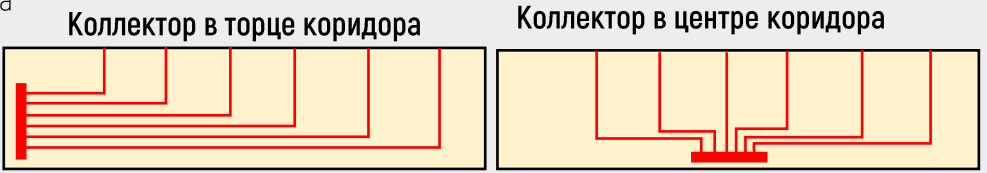
Длина трубопроводов: L1 = 150 метров L2 = 90 метров. Разница 70%
