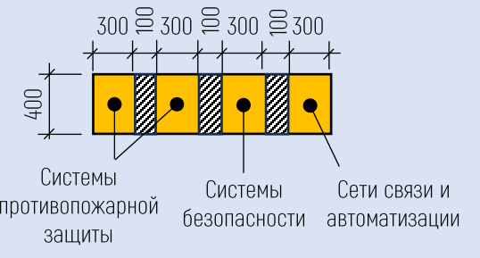
Шахты для транзитных общедомовых систем
